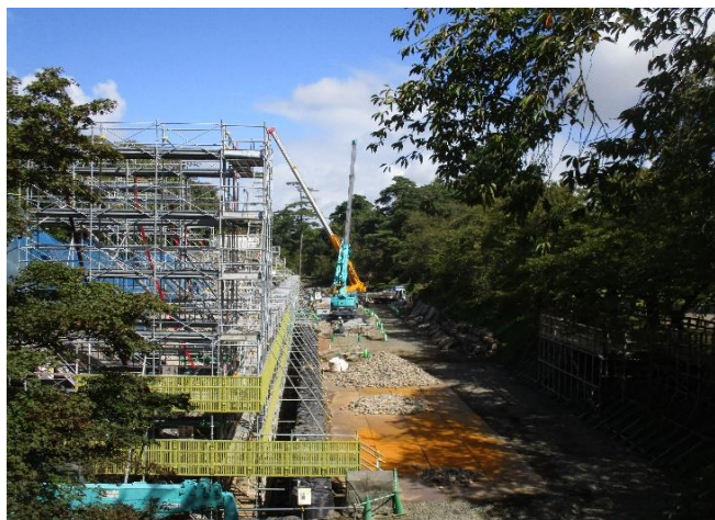
下乗橋から工事現場を望む（令和3年9月13日撮影）
