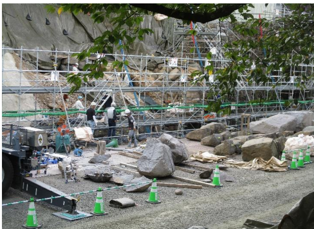
石垣積直し・新補石加工
