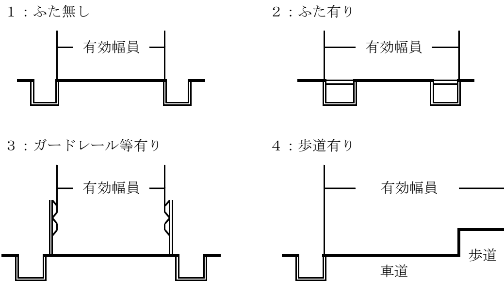
図1 道路の有効幅員（第12条第1項第4号関係）
