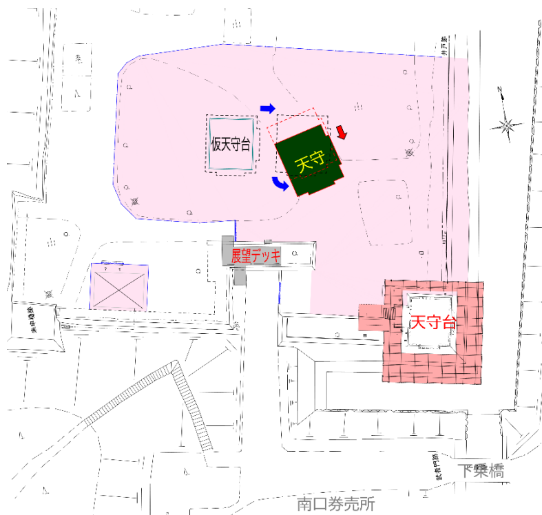
令和8年9月15日時点の天守位置 【二次移動中（一次移動先から4.67m南へ移動）】
